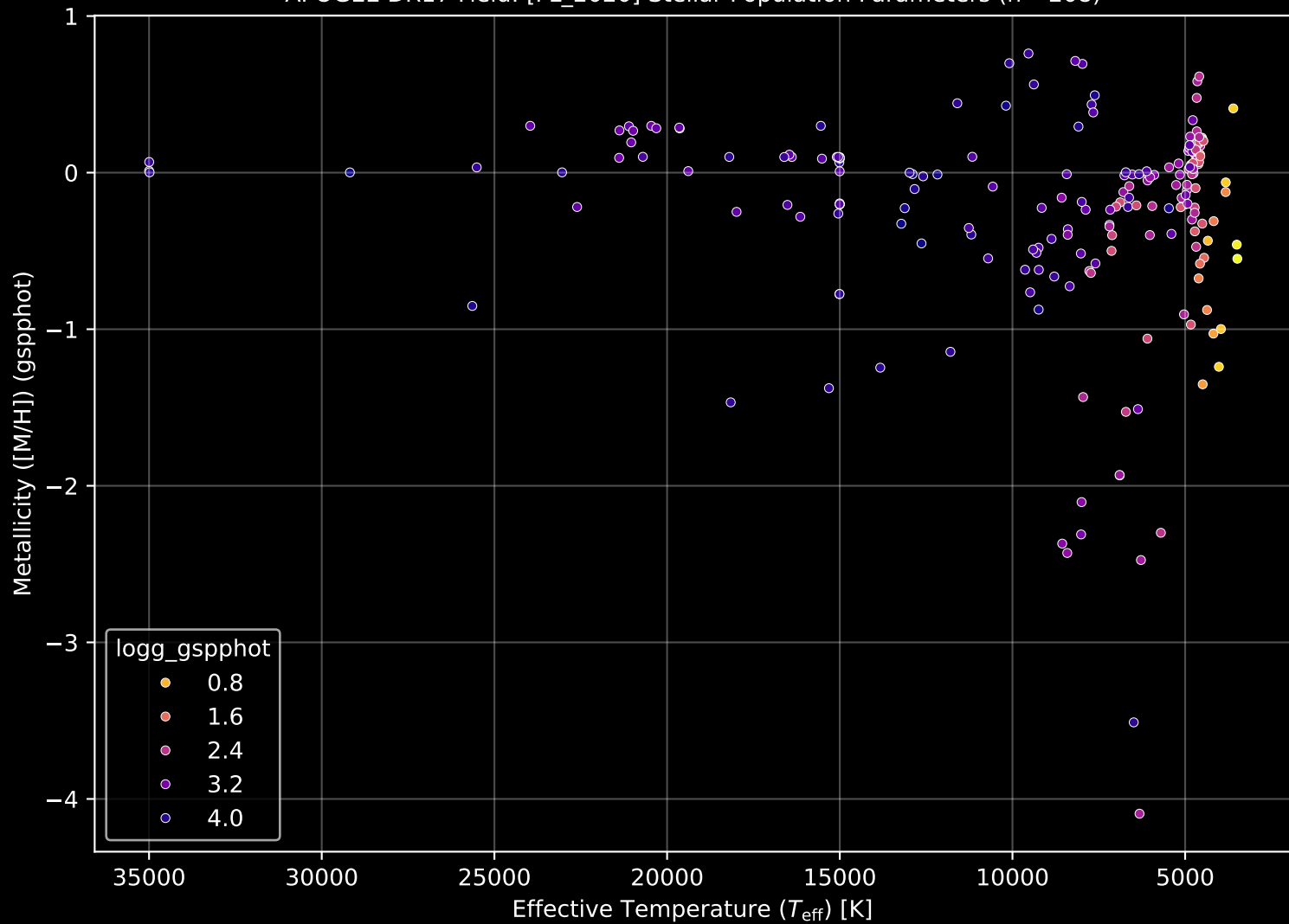
APOGEE DR17 Field: [FL_2020] Stellar Population Parameters (n= 208)
